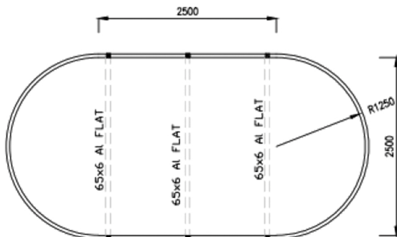
PLAN SCALE 1 : 50
